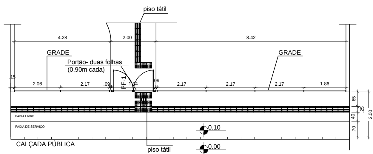
Detalhe de Grade, Portão e Calçada Pública
