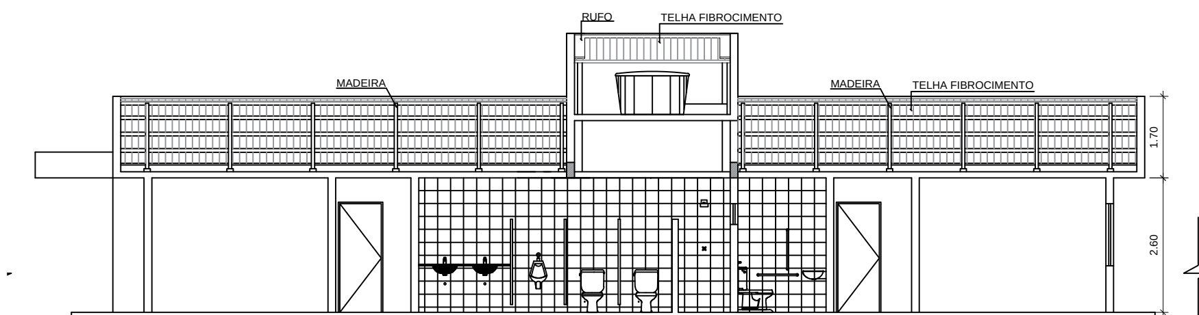
CORTE C-C
