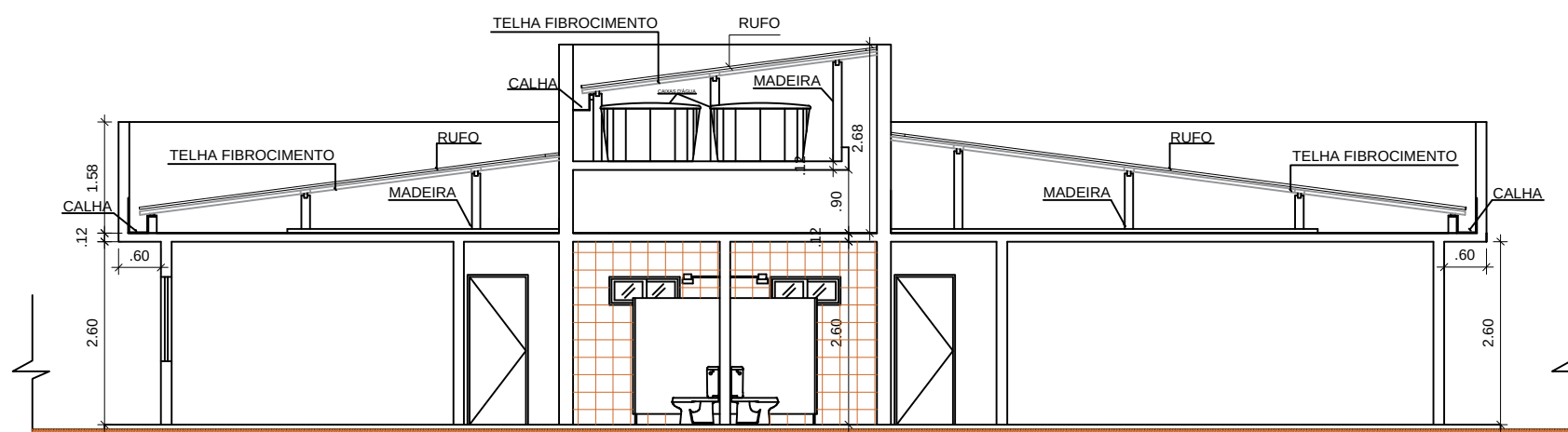
CORTE A-A
