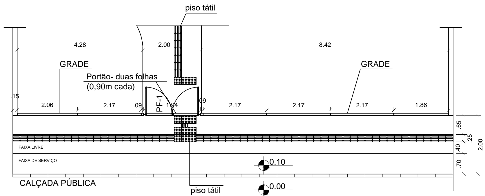
Detalhe de Grade, Portão e Calçada Pública
