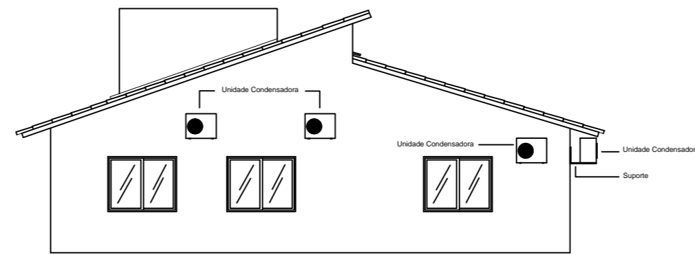
FACHADA POSTERIOR
