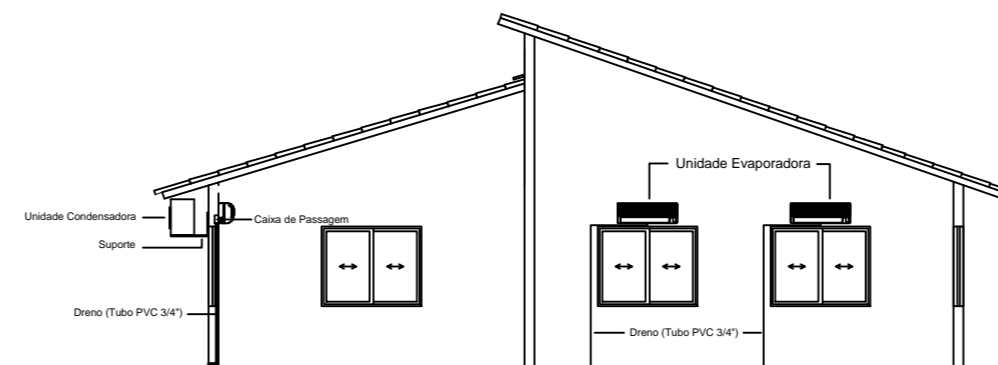
CORTE A-A
