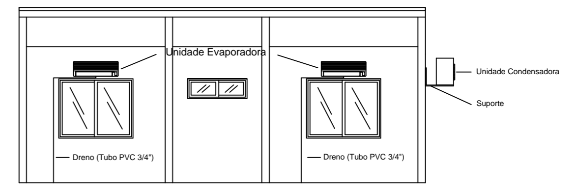
CORTE A-A
