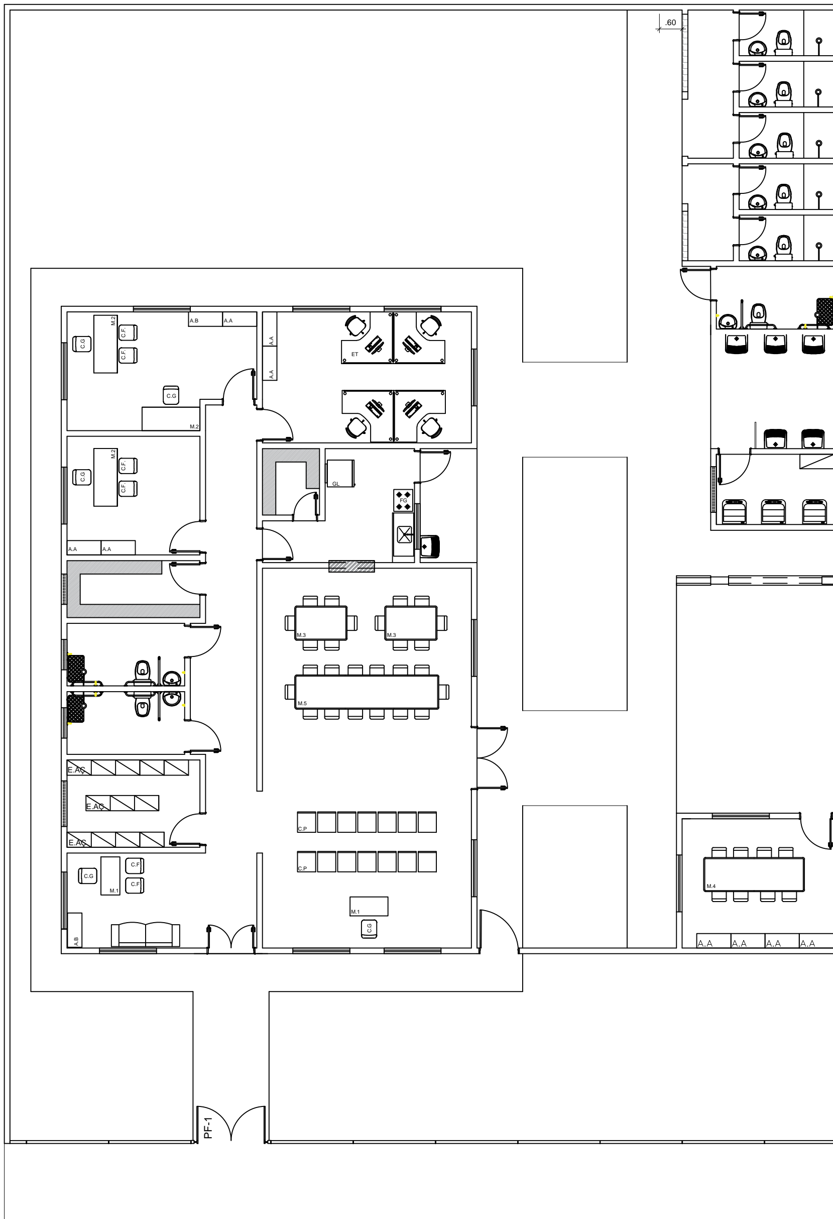
PLANTA DE LAYOUT ESCA 1:100
