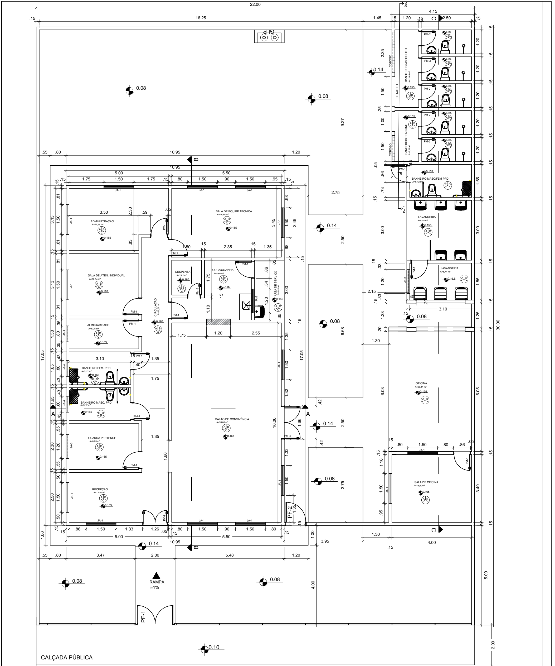
PLANTA BAIXA ESCALA 1:100
