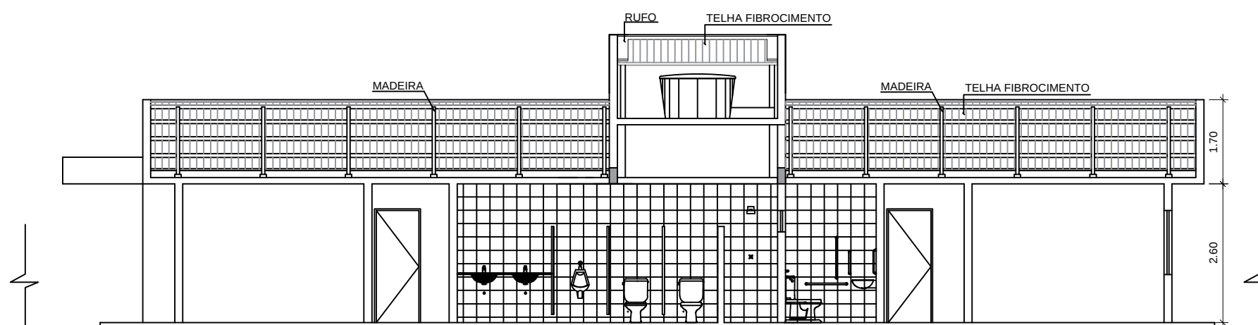
CORTE C-C
