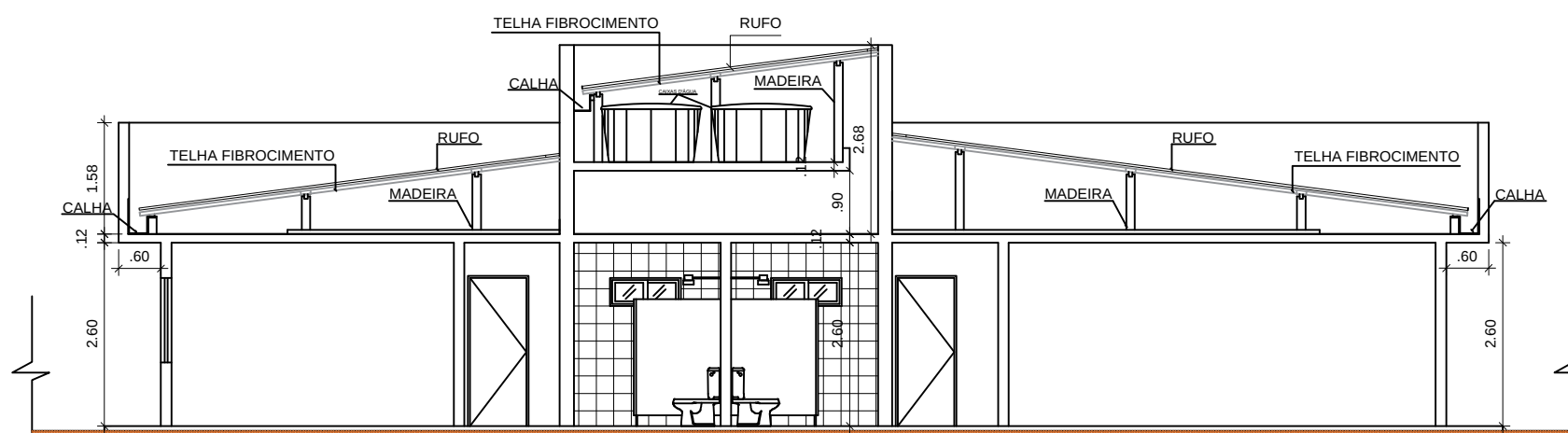
CORTE A-A
