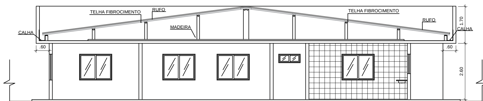
CORTE B-B
