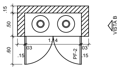
DETALHE ABRIGO GLP :
