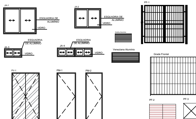
DETALHE DE ESQUADRIAS
