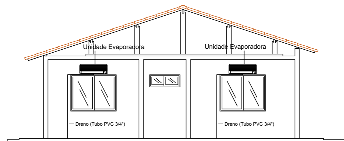
CORTE A-A
