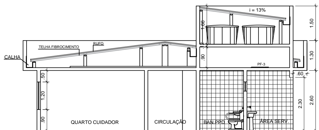
CORTE B-B
