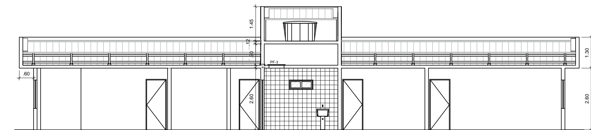
CORTE C-C
