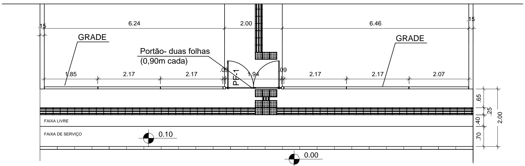
Detalhe de Grade, Portão e Calçada Pública
