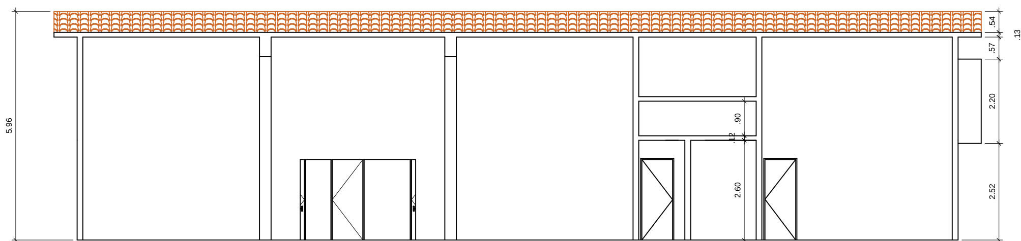
CORTE C-C
