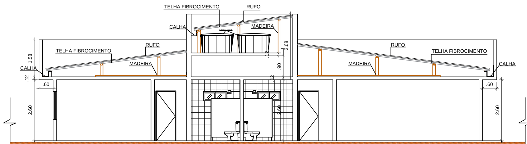
CORTE A-A
