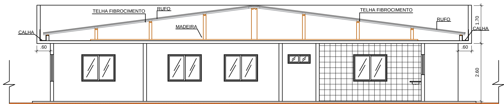
CORTE B-B
