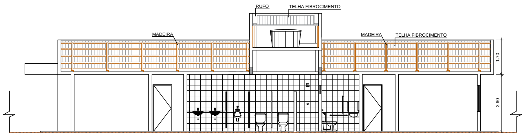
CORTE C-C
