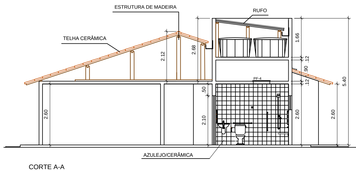
CORTE A-A
