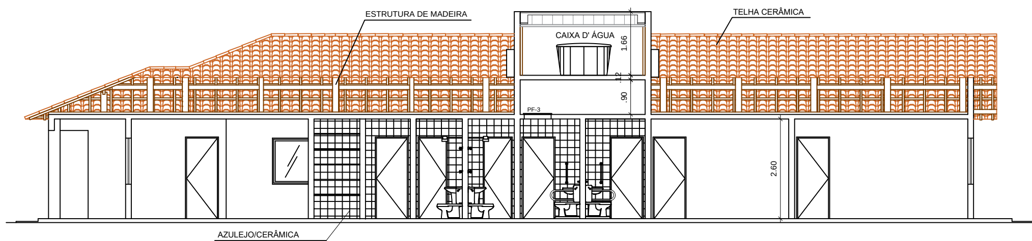
CORTE B-B
